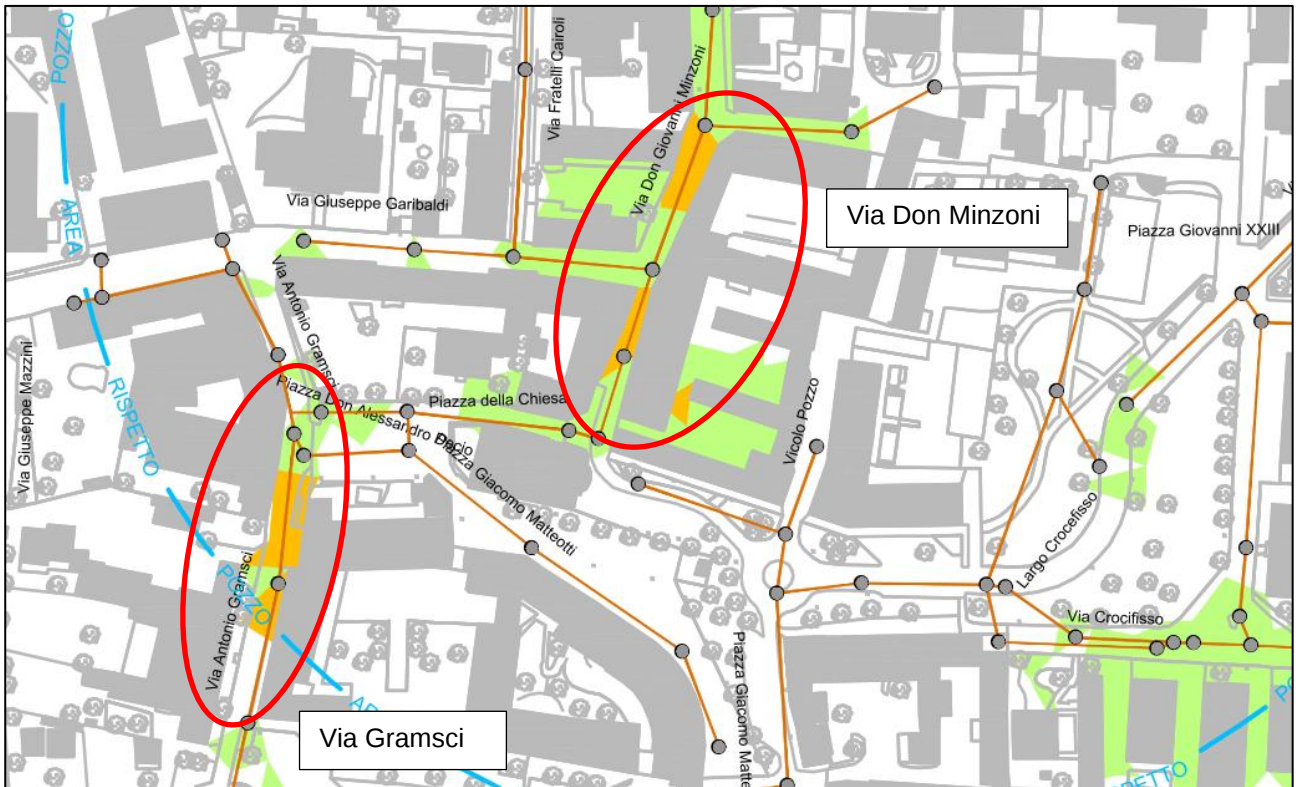
Figura 2: Aree con criticità idraulica T50 in Via Gramsci e Via Don Minzoni
