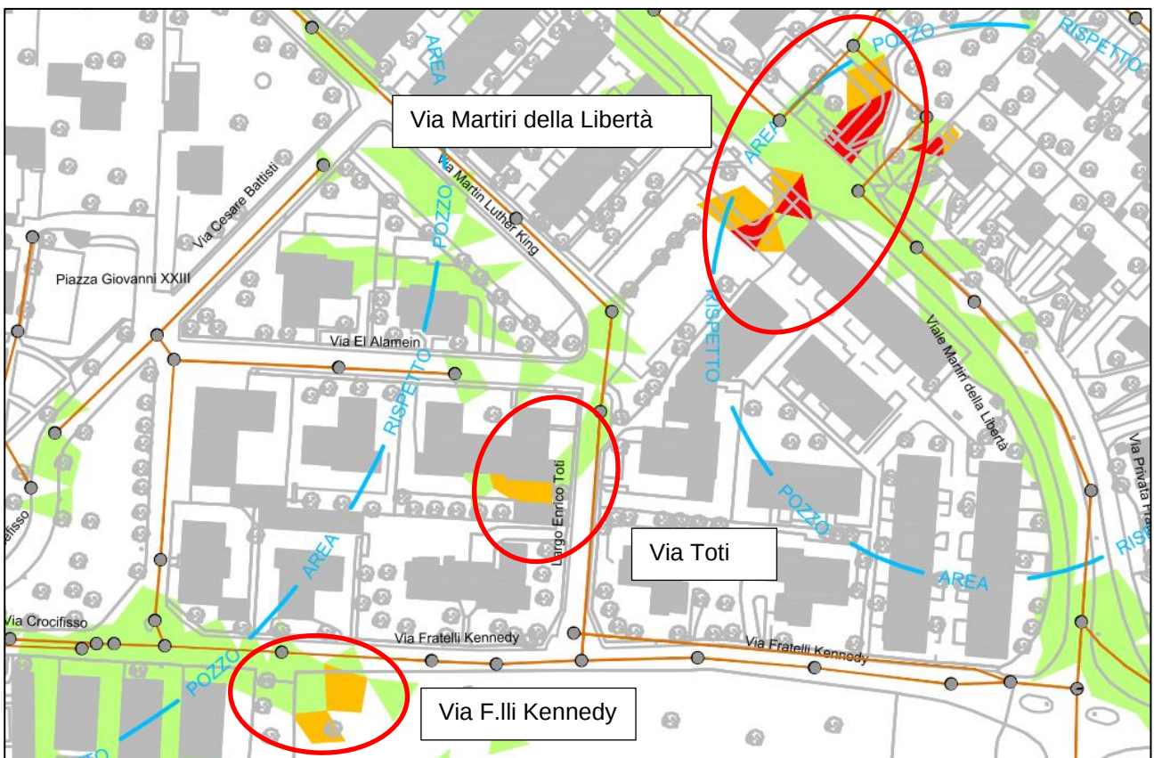
Figura 3: Aree con criticità idraulica T50 in Via Martiri della Libertà, Via Toti e Via F.lli Kennedy
